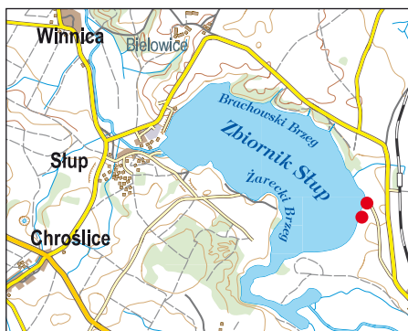
Ryc. 5. Rozmieszczenie Cucubalus baccifer .
