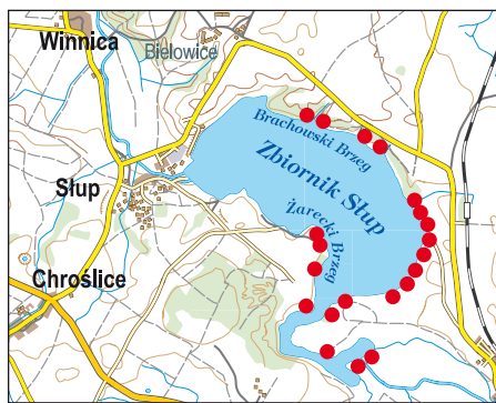
Ryc. 8. Rozmieszczenie Isolepis setacea . Fig. 8. Distribution of Isolepis setacea .
