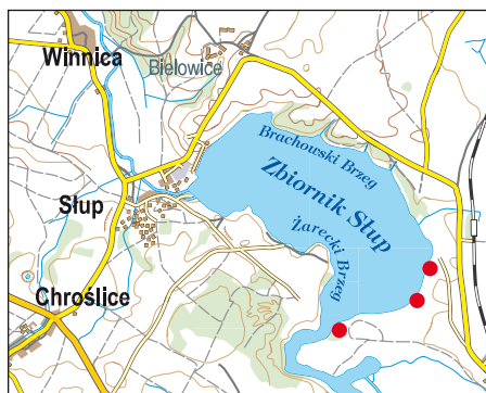
Ryc. 6. Rozmieszczenie Cyperus fuscus .
