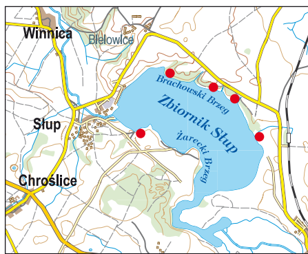
Ryc. 12. Rozmieszczenie Vulpia myuros . Fig. 12. Distribution of Vulpia myuros .
