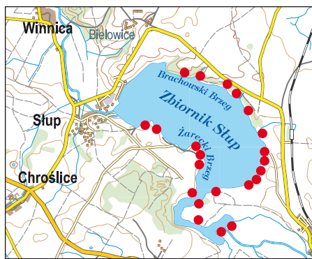
Ryc. 10. Rozmieszczenie Limosella aquatica . Fig. 10. Distribution of Limosella aquatica .
