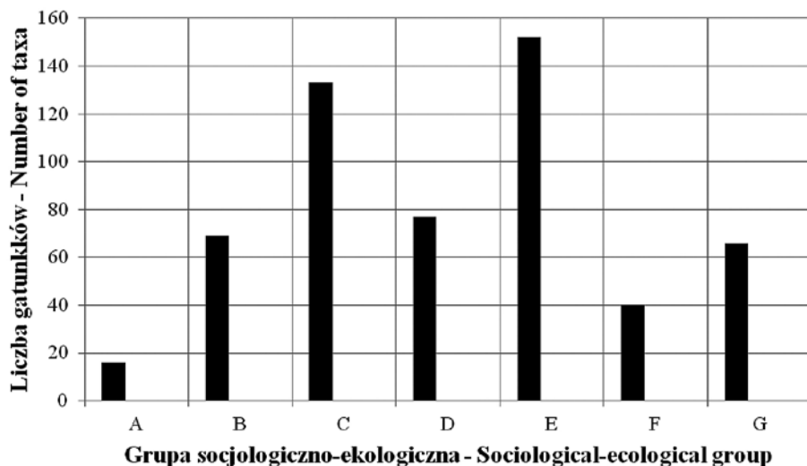
Ryc. 15. Grupy socjologiczno-ekologiczne flory naczyniowej zbiornika retencyjnego Słup.
