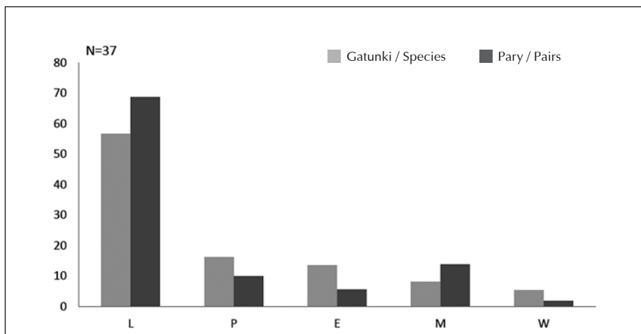
Ryc. 2. Procentowy udział gatunków oraz ich liczebność pod względem kategorii siedliskowej: L – gatunki leśne, P – ptaki otwartego krajobrazu, E – ptaki ekotonu, M – gatunki synantropijne, W – ptaki związane ze środowiskiem wodnym.
