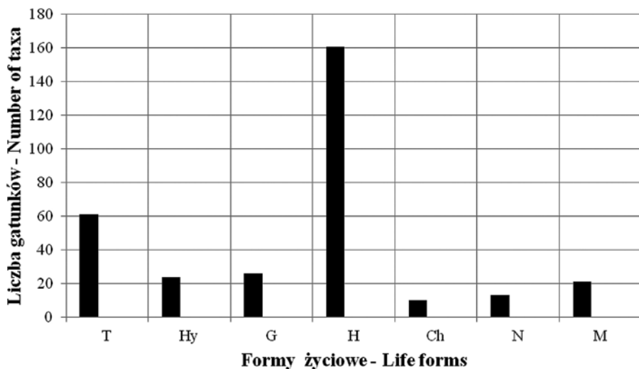
Ryc. 13. Formy życiowe roślin naczyniowych zbiornika retencyjnego Słup.
