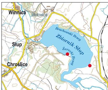
Ryc. 9. Rozmieszczenie Leersia oryzoides . Fig. 9. Distribution of Leersia oryzoides .
