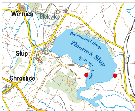
Ryc. 11. Rozmieszczenie Schenoplectus tabernaemontani . Fig. 11. Distribution of Schenoplectus tabernaemontani .
