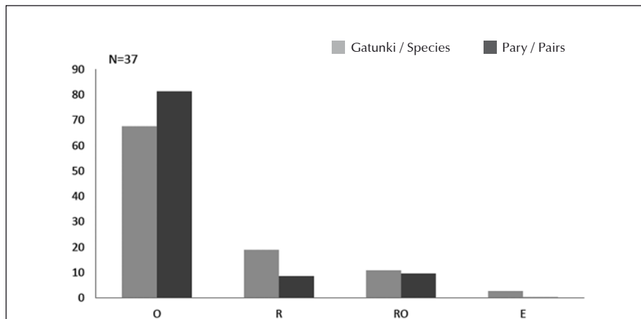
Ryc. 3. Procentowy udział gatunków oraz ich liczebność pod względem kategorii pokarmowej: O – owadożerne, R – roślinożerne, RO – o pokarmie mieszanym (roślinno-owadzi), E – euryfagi.
