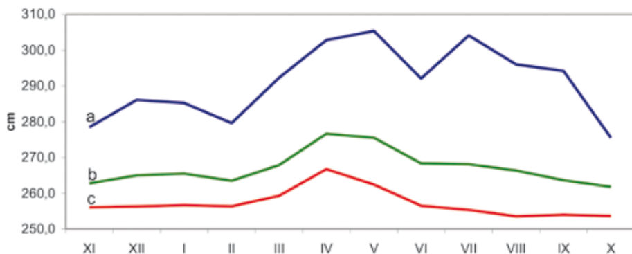
Ryc. 4. Miesięczne wartości stanów wody w okresie 1961-2010: a) średnie maksymalne, b) średnie, c) średnie minimalne.
