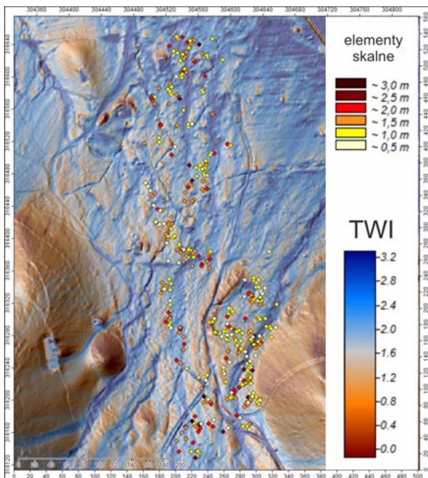
Ryc. 4. Rozmieszczenie dużych elementów skalnych na powierzchni stożka (dolina 3), skala topograficznego indeksu wilgotności (TWI) jest niemianowana.
