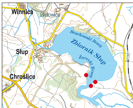
Ryc. 7. Rozmieszczenie Eleocharis ovata . Fig. 7. Distribution of Eleocharis ovata .
