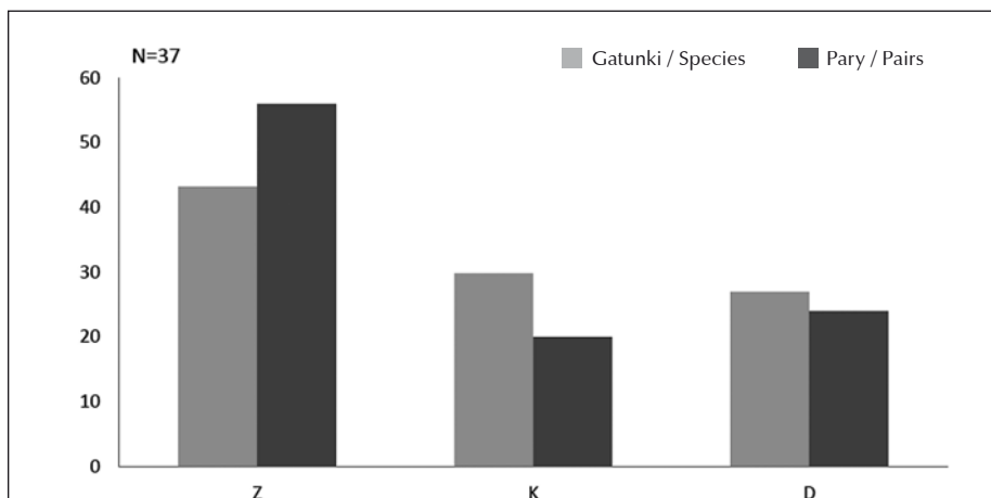
Ryc. 4. Procentowy udział gatunków oraz ich liczebność pod względem kategorii gniazdowej: Z – gniazdujące na ziemi lub tuż nad ziemią (do wysokości 1,5 m), albo na wodzie, K – gniazdujące w koronach krzewów i drzew, D – dziuplaki.
