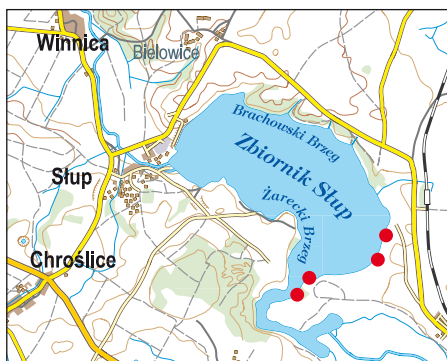
Ryc. 3. Rozmieszczenie Carex bohemica .
