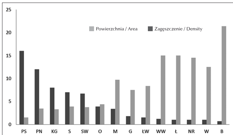
Ryc. 5. Wpływ całkowitej powierzchni badanych kamieniołomów na zagęszczenie zespołów awifauny.
