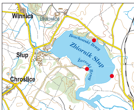
Ryc. 1. Rozmieszczenie Allium angulosum .
