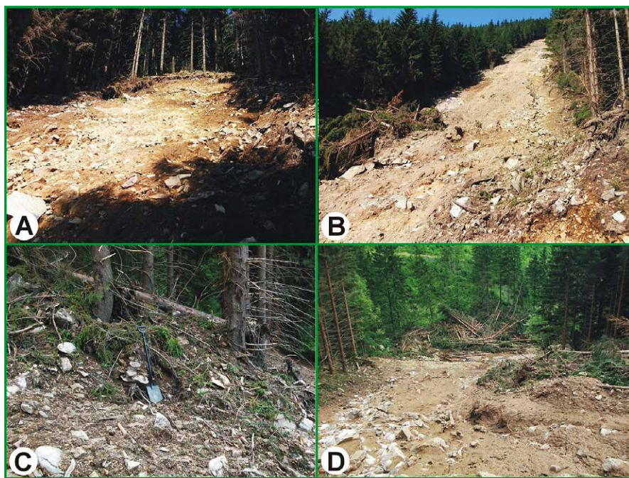
Fot. 2. Główne elementy rzeźby w obrębie osuwiska na Średniaku. A. Strefa oderwania mas skalnych, B. Rzeźba osuwiska zajmująca największe powierzchnie: odsłonięte podłoże skalne z cienką pokrywą rezydium zwietrzliny rozcinanej przez wody odpływające ze źródeł (oznaczonych sygnaturą), C. wał akumulacyjny w brzeżnej części osuwiska, D. strefa akumulacyjna osuwiska: na pierwszym planie koluwia, w dali nagromadzenie rumoszu drzewnego (fot. K. Parzóch).
