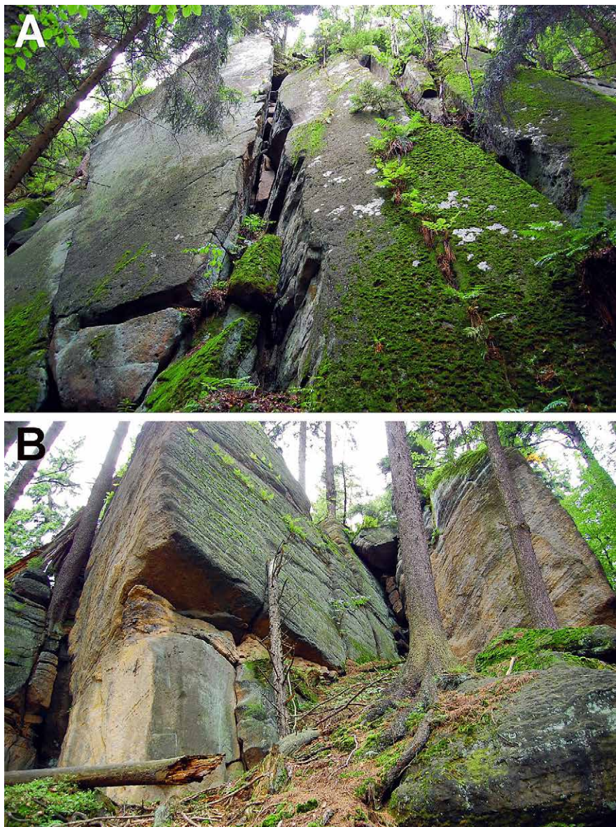
Fot. 1. Ściana skalna w górnym odcinku progu Gór Stołowych pod Białą Skalą. A – odcinek o przebiegu prostym, B – odcinek o przebiegu klinowym, nawiązującym do krzyżujących się zespołów spękań (fot. M. Kasprzak).
