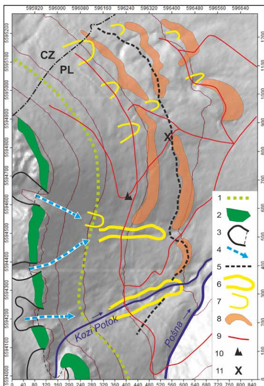
Ryc. 7. Szkic morfologiczny progu Gór Stołowych pod Białą Skałą.
