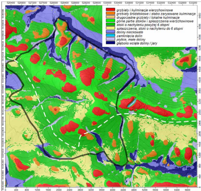
Ryc. 12. Mapa głównych form rzeźby (parametr TPI). Poligonem oznaczono obszar analizy geomor- fometrycznej. Biała linia określa granicę między granitem karkono- skim a metamorfikiem izerskim.
