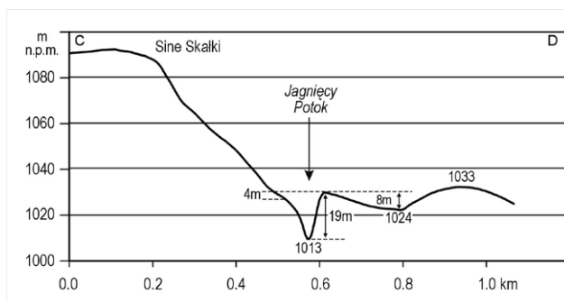
Ryc. 7. Profil morfologiczny w poprzek górnego odcinka doliny Jagnięcego Potoku. Jar o głębokości do 19 m jest odsunięty od równoległego, słabiej wykształconego obniżenia (pomiar wysokości względnych na podstawie DEM).
