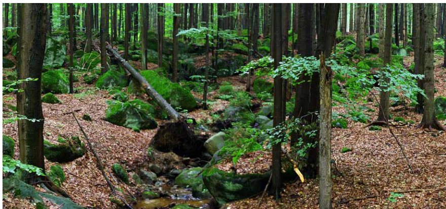
Fot. 4. Strumień głazowo-blokowy w dolinie Koziego Potoku, przemywany przez potok (fot. M. Kasprzak).
