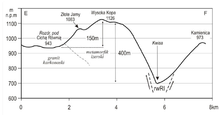
Ryc. 5. Profil morfologiczny przez zachodnią część masywu Zielonej Kopy. Objaśnienia: rwRI – rów Rozdroża Iżerskiego, liniami przerywanymi oznaczono hipotetyczne linie dyslokacji tektonicznych, schematyczne granice litologiczne na podstawie przekrojów geologicznych zamieszczonych na SzMGS 1:25 000 (arkusze Rozdroże Iżerskie, Świeradów Zdrój).
