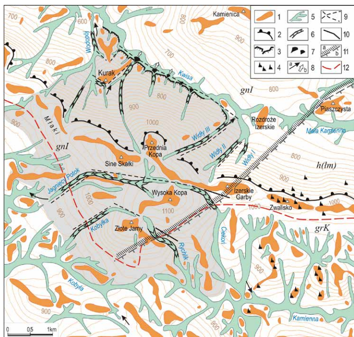
Ryc. 14. Mapa wynikowa prezentująca główne cechy rzeźby w aspekcie analizy uwarunkowań strukturalnych i tektonicznych. Objaśnienia: 1 – grzbiety i ostańce denudacyjne, 2 – załom wypukły ograniczający od północy wierzchołkę Grzbietu Wysokiego, 3 – skarpy morfologiczne (uskokowe), 4 – skałki, 5 – dna dolin, 6 – wciśnięte (jarowe) odcinki dolin, 7 – stożki napływowe, 8 – przypuszczalne kierunki dawnych przepływów (a), kierunku bocznej migracji koryta Kwisy (b), 9 – przypuszczalne uskoki, 10 – uskoki wyznaczone na SzMGS, 11 – schematyczny przebieg żyły kwarcowej (a), nasunięcie Rozdroża Iżerskiego (b), 12 – granica między granitem karkonoskim a metamorfikiem iżerskim; grK – granit karkonoski, h(lm) – hornfelsy i łupki metamorficzne, gnI – gnejsy i granity iżerskie.
