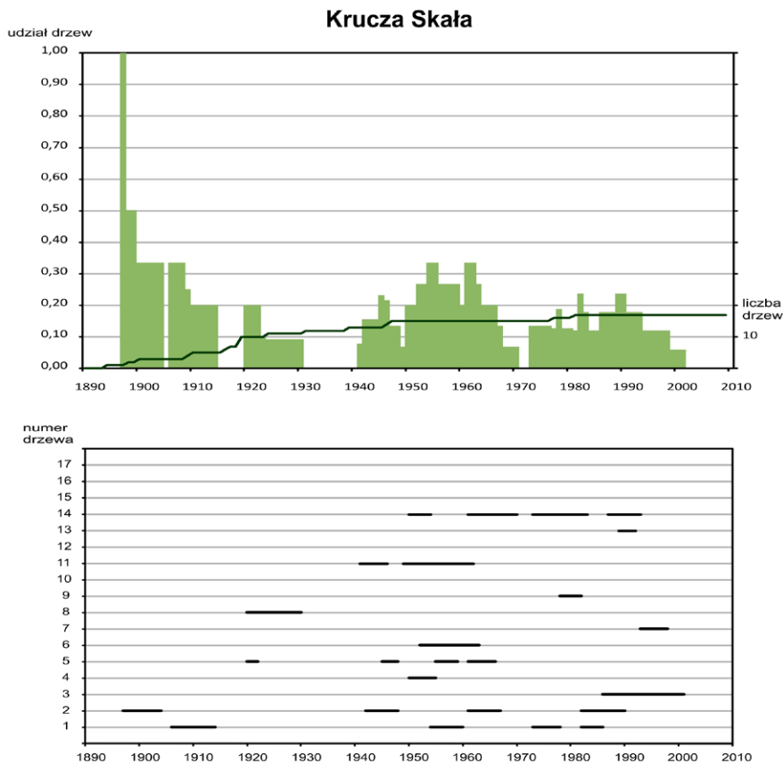
Ryc. 4. Krucza Skała. Udział drzew wykształcających w danym roku dekoncentryczny przyrost (słupki) w całkowitej liczbie opróbowanych drzew (linia) (góra) oraz okresy wytwarzania przez poszczególne drzewa drewna reakcyjnego (dół).
