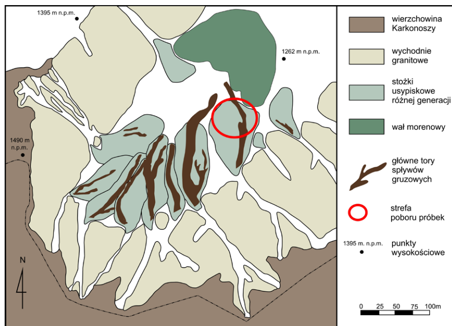
Ryc. 1. Szkic morfologiczny Wielkiego Śnieżnego Kotła w Karkonoszach z oznaczeniem głównych rynien sypwów gruzowych w obrębie stożków usypiskowych (według: MICOŃ i in. 2010).
